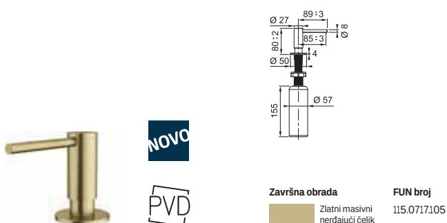
DOZATOR TEČNOG DETERDŽENTA ATLAS
